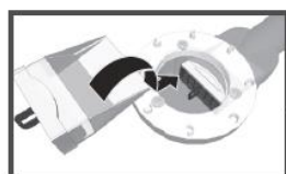
MEMBRANA Y FILTRO accesibles por encima
